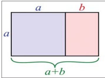
رسم بياني للمستطيل الذهبي، الذي ينتج عن قسمة ابعاد اضلاع- النسبة الذهبية (phi)
