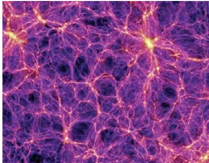
• المادة المظلمة ليست كل الحقيقة
