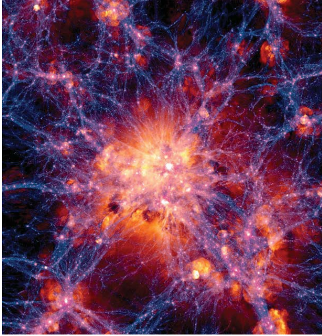
المادة المظلمة والمادة المظلمة وإعادة إنتاج الكون
