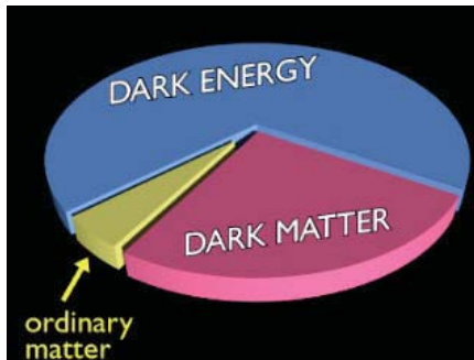
• اللون الأزرق يشير إلى حجم الطاقة المظلمة والرمزي للمادة المظلمة أما الأصفر فهو المادة الاعتيادية
